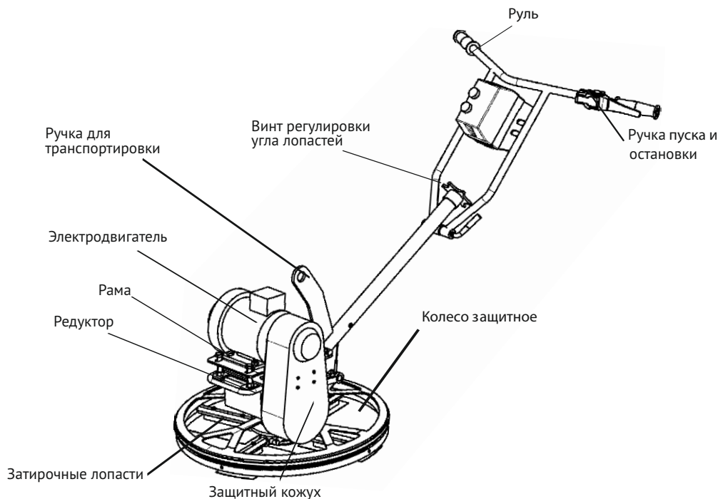
Рис. 1 Общий вид машины WIPE T600
